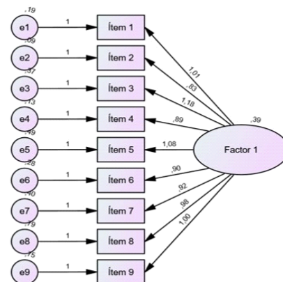
Figura 2. Análisis factorial confirmatorio de la escala de actitudes negativas hacia personas trans.
