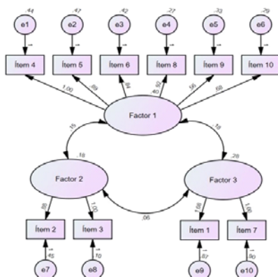
Figura 1. Análisis factorial confirmatorio de la escala de homofobia EHF-10.
